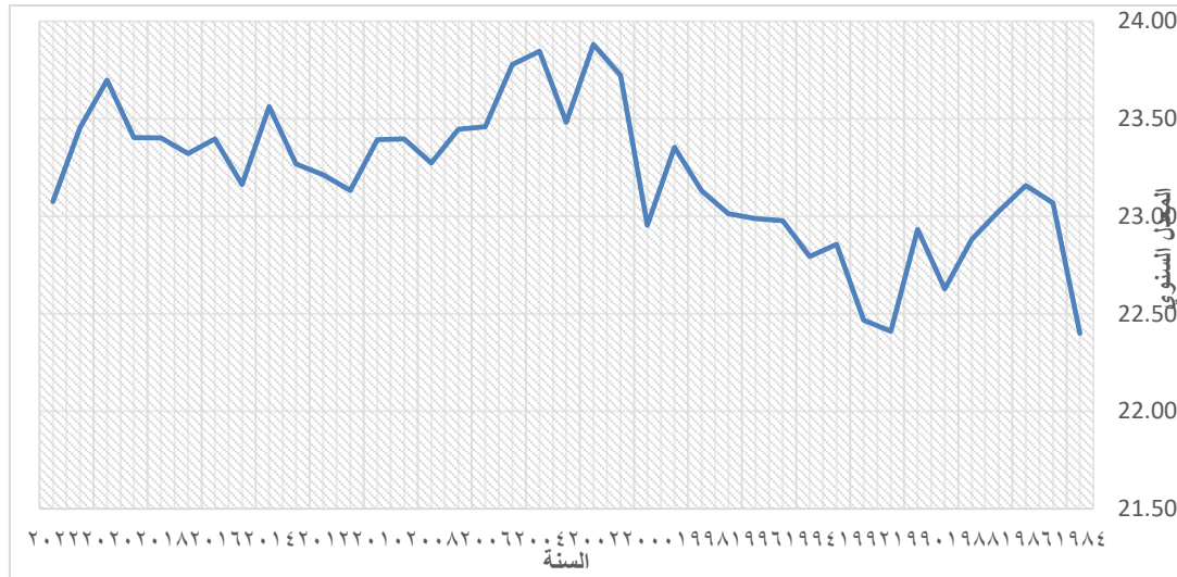
شكل ٤. المعدل السنوي للإشعاع الشمسي بمحافظه القنفذه من عام (١٩٨٤م - ٢٠٢٢م).
